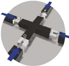
Соединение при помощи X-коннектора
